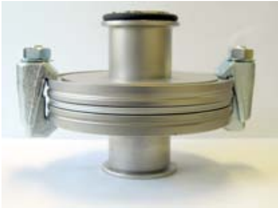
fig. 135: ISO-K flange (middle)
